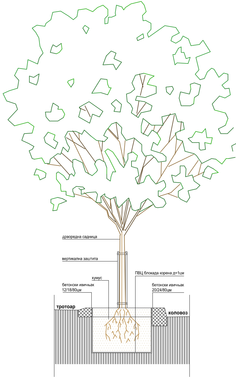
Пресек 1-1
